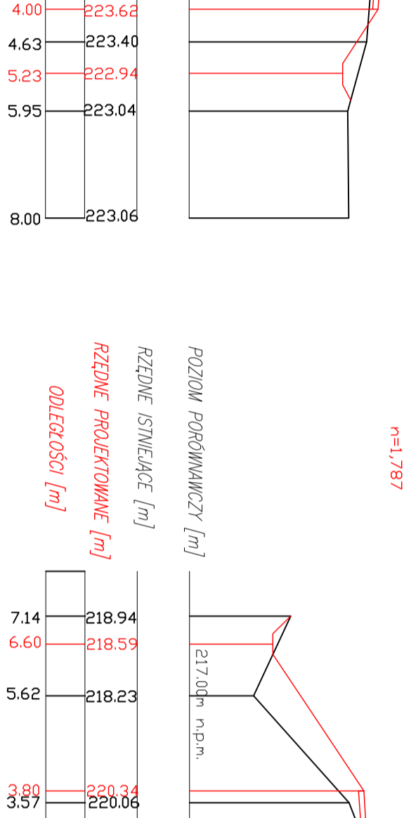
Przekrój poprzeczny nr 33 km 1+572,45
