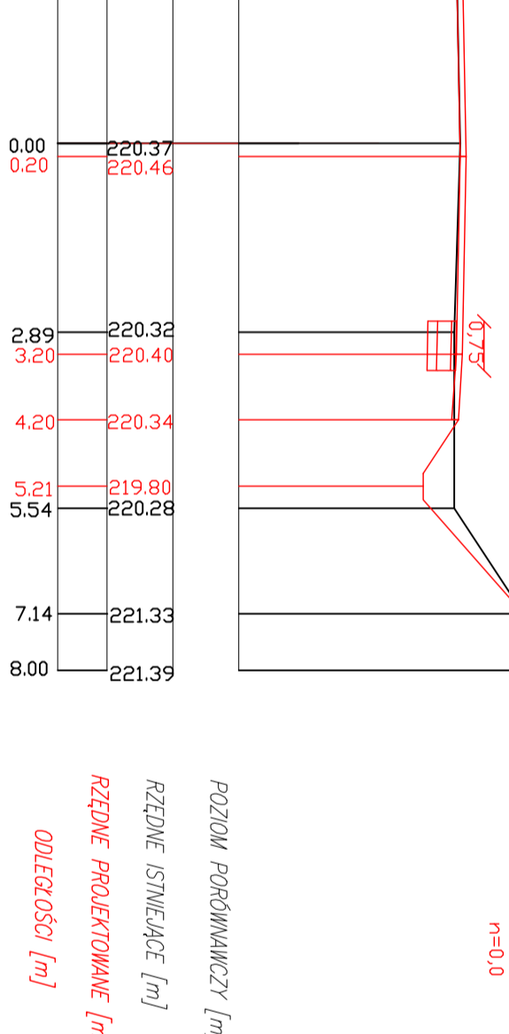
Przekrój poprzeczny nr 34 km 1+621,21
