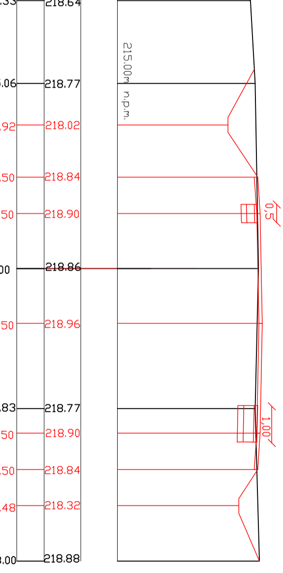
Przekrój poprzeczny nr 35 km 1+665,86
