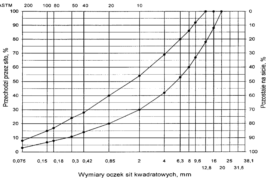
Rys. 9. Krzywe graniczne uziarnienia mieszanek mineralnej BA od 0 do 16 mm do warstwy wiążącej, wyrównawczej i wzmacniającej nawierzchni drogi o obciążeniu ruchem KR1 lub KR2
